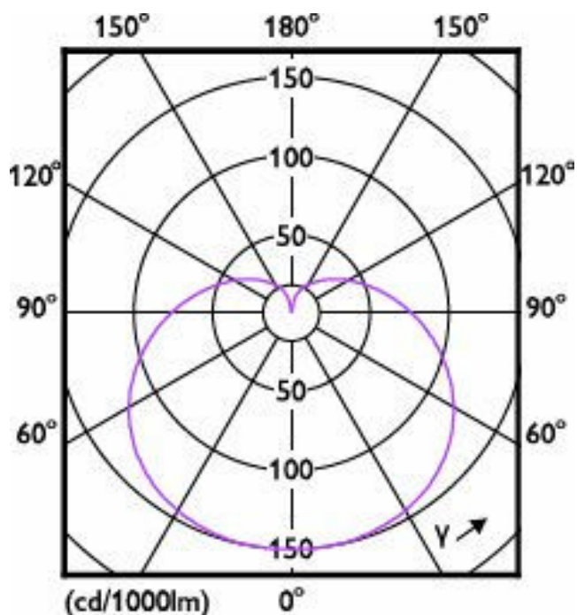
Light Distribution Diagram - LEDBulb 9W E27 DS FR DIM 1PF/6 AU
