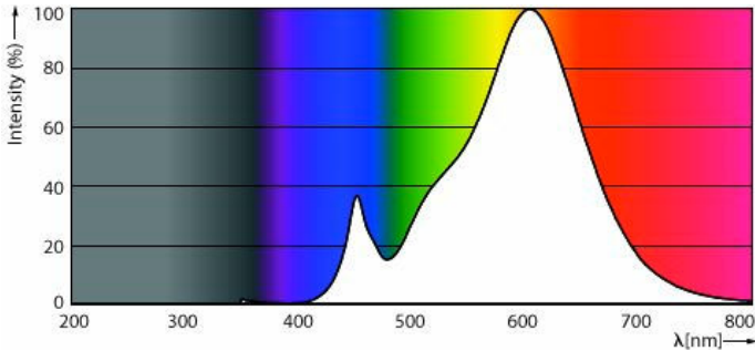
Spectral Power Distribution Colour - LEDBulb 9W E27 DS FR DIM 1PF/6 AU
